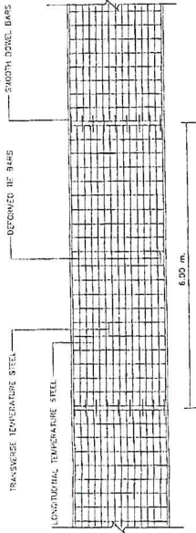
แบบโครงสร้างทางคอนกรีตเสริมเหล็ก ๓.๕๐
